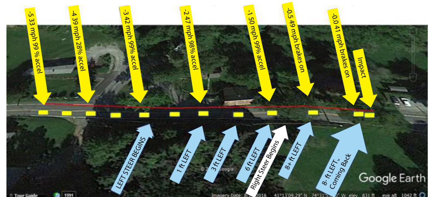
Slika 6: Primer uporabe diagrama, ki prikazuje pot vozila, pospeševanja, zaviranja, spremembe hitrosti in zavijanja krmila (Vir: Peters, 2019)
