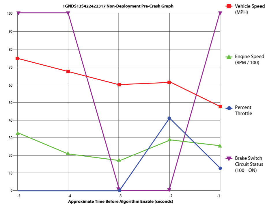
Slika 8: Parametri vozila pred trčenjem (hitrost vozila, število obratov motorja, uporaba stopalke za plin in zaviranje)
