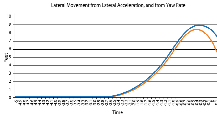
Slika 7: Graf prevožene bočne poti vozila B glede na časovne intervale pred trčenjem (modra krivulja prikazuje izračunano pot na podlagi delovanja sile pospeška, oranžna pa izračun glede na vrednost zanašanja vozila) (Vir: Ruth, 2019)
